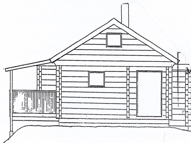
Fasad Syd-väst
