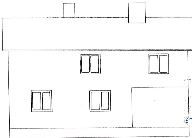
FASAD MOT ÖSTER SKALA 1:100
