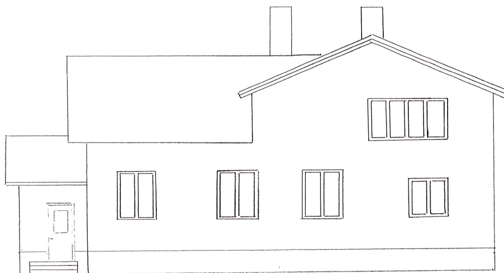
FASAD MOT SÖDER SKALA 1:100
