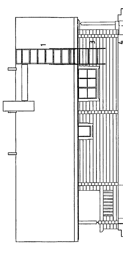
Julkisivu 3
